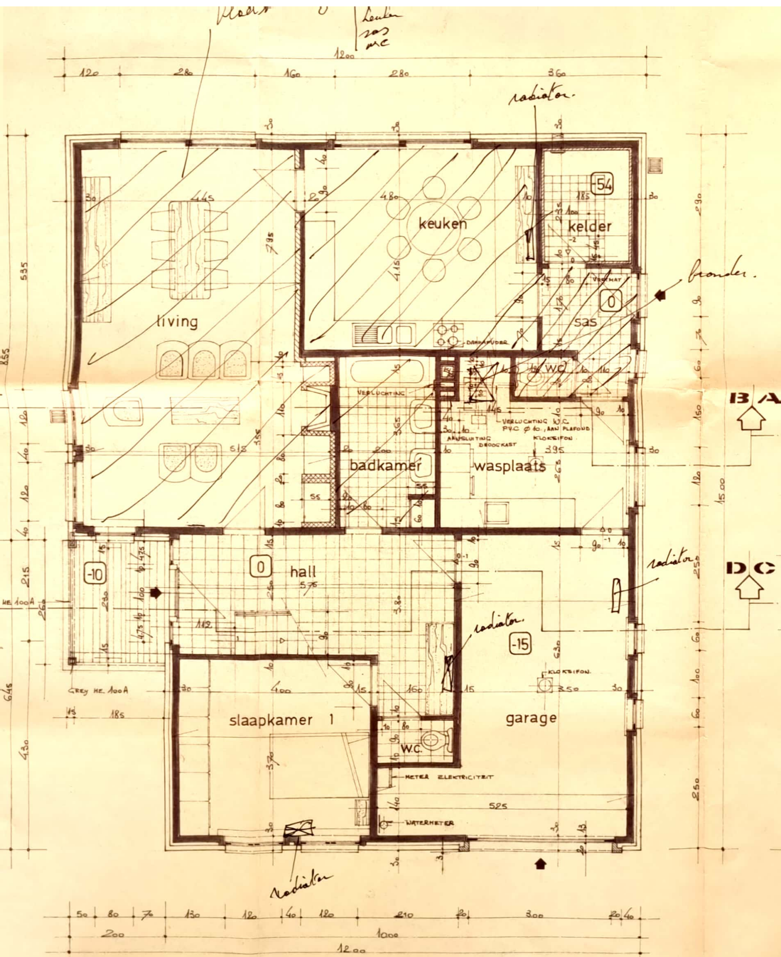
grondplan
